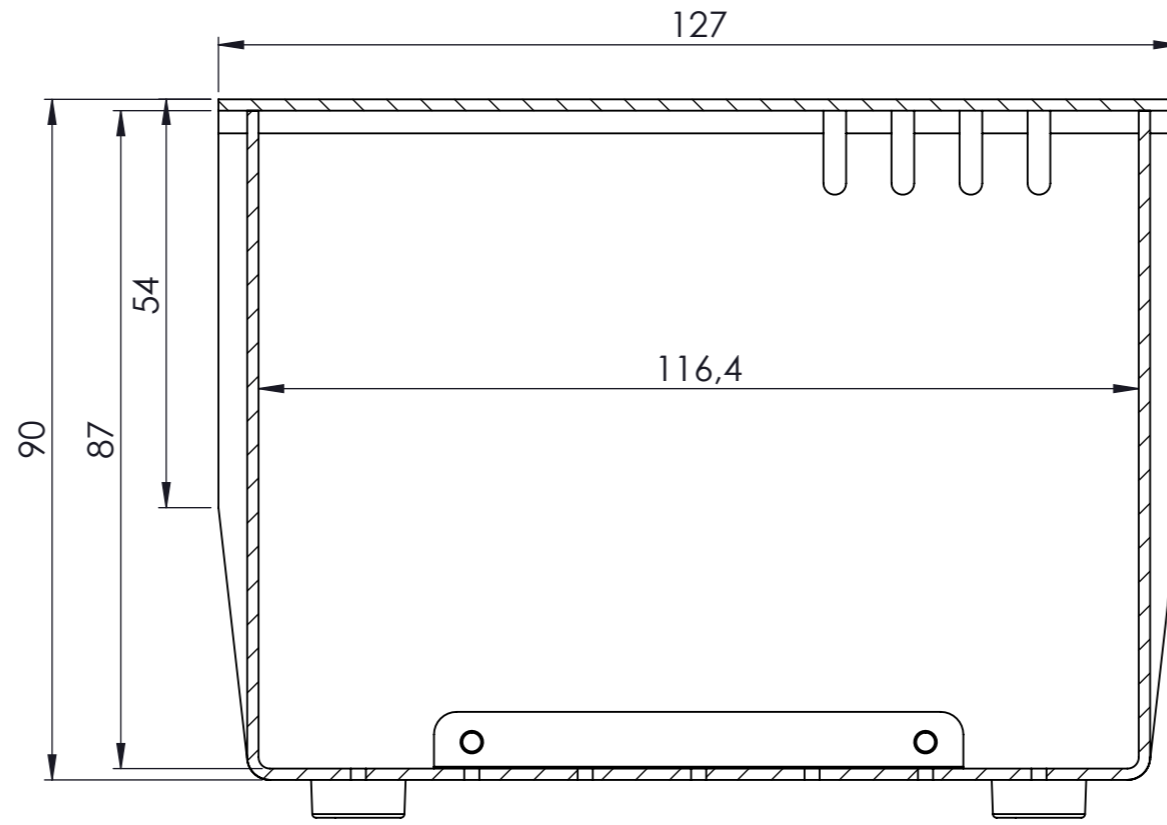
KESIT A-A
