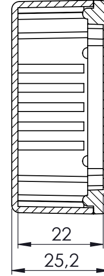
KESIT A-A
