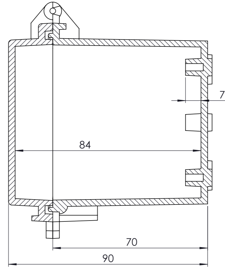
KESIT A-A
