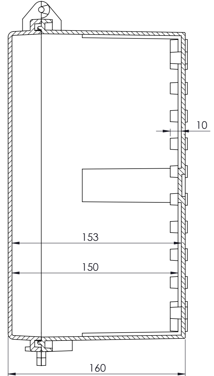
KESIT A-A
