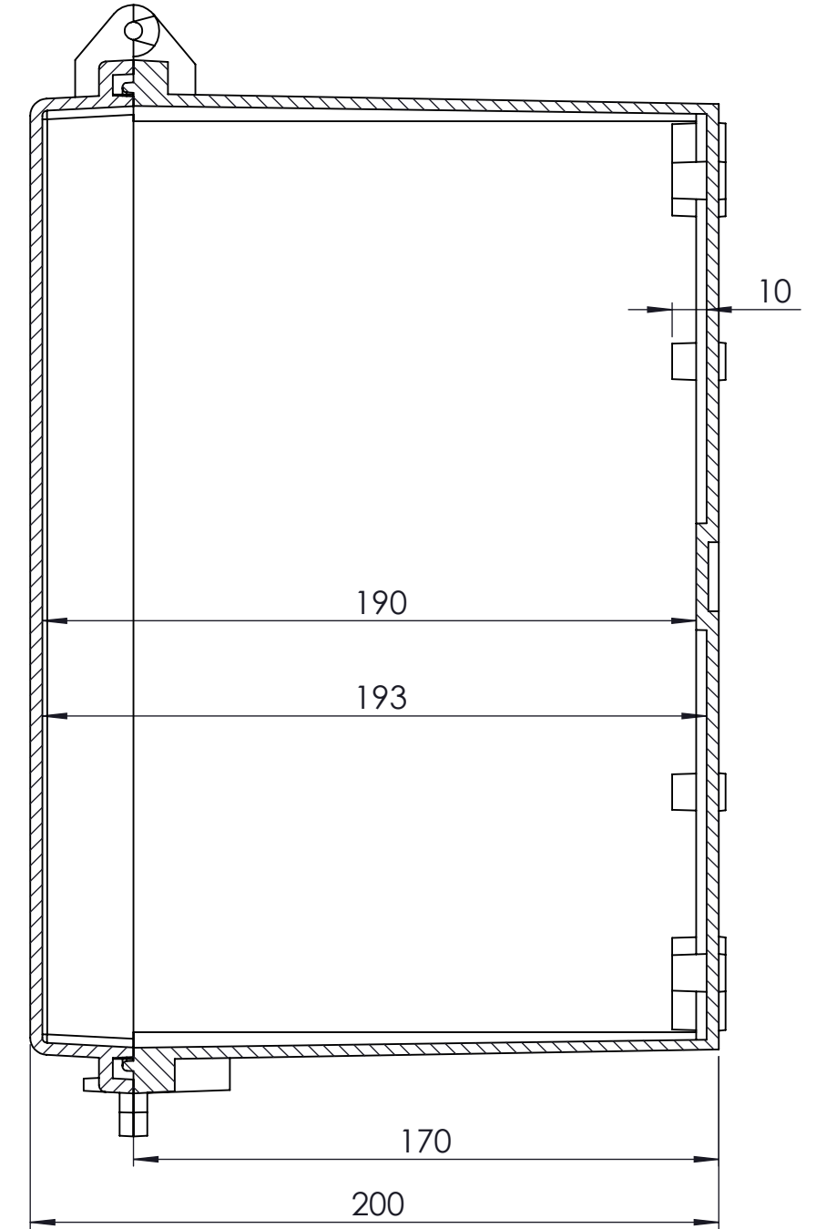
KESIT A-A
