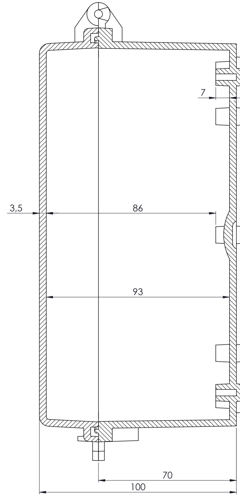
KESIT A-A
