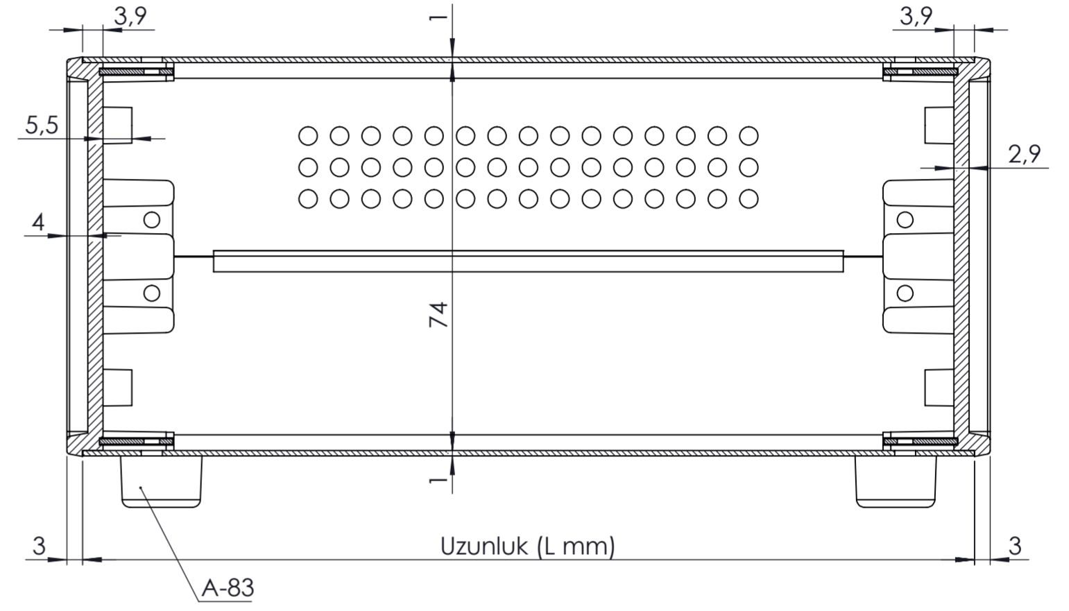
KESIT A-A
