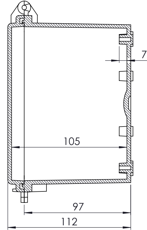
KESIT A-A
