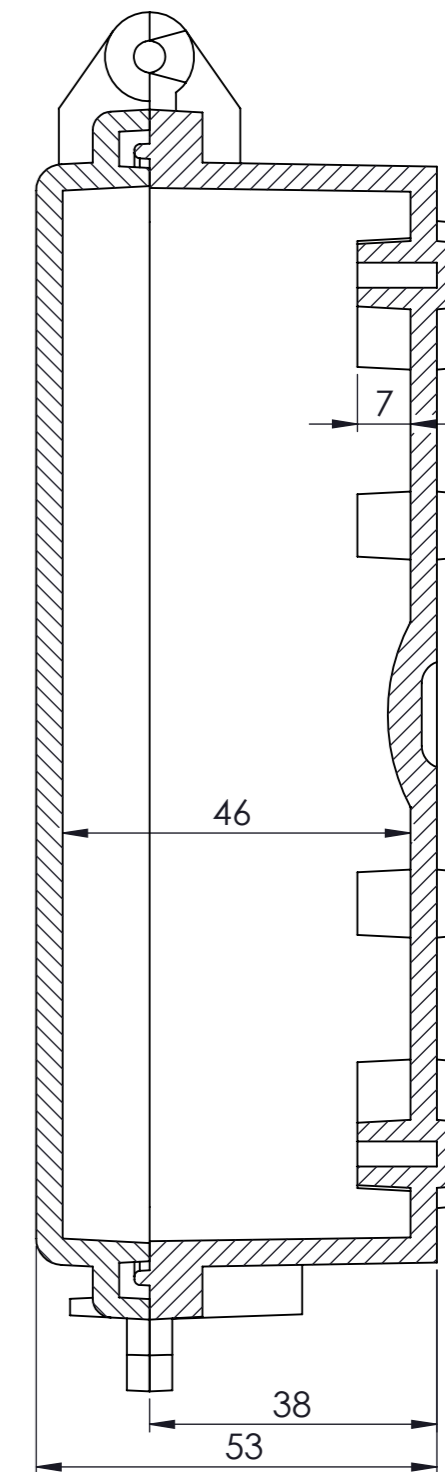
KESIT A-A
