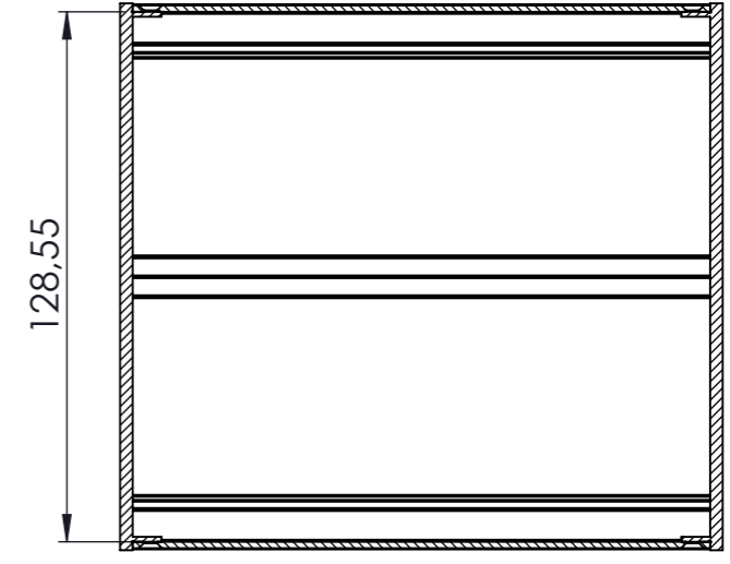
KESIT A-A
