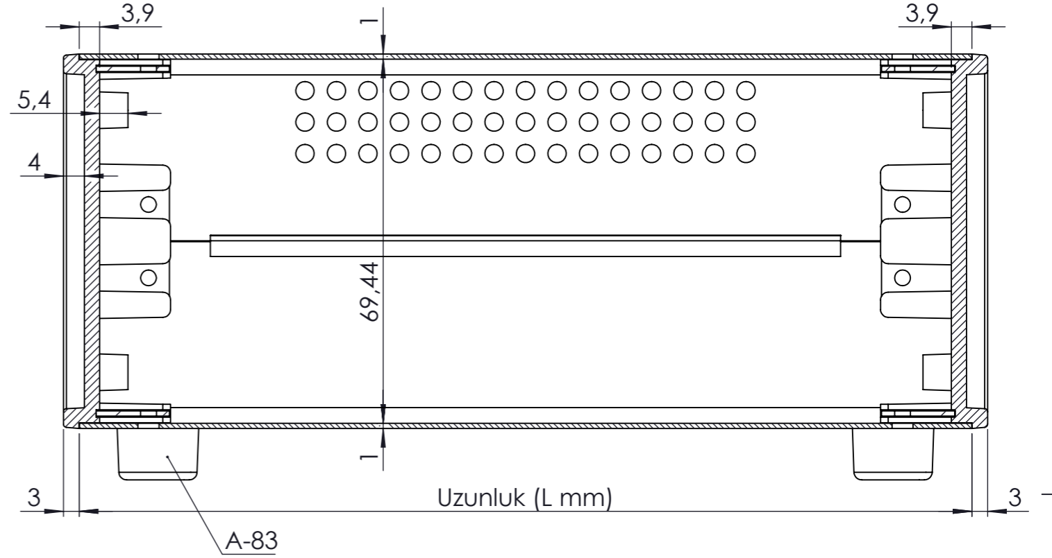
KESIT A-A
