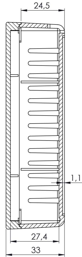
KESIT A-A
