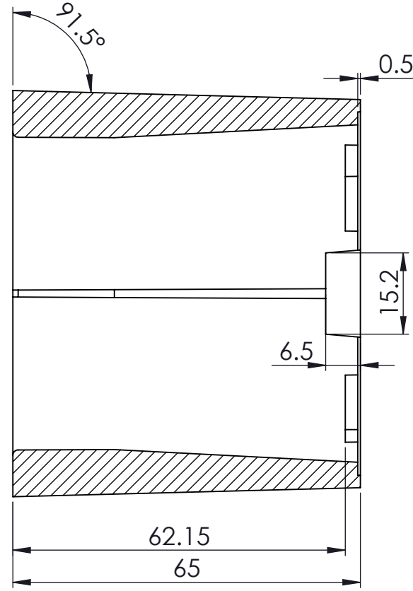
KESIT A-A
