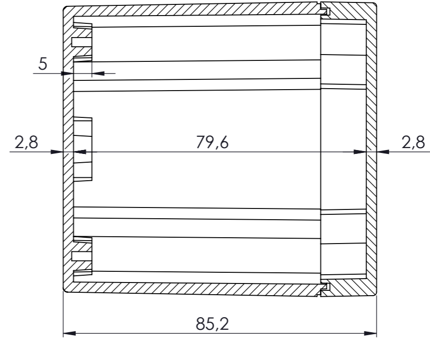
KESIT A-A
