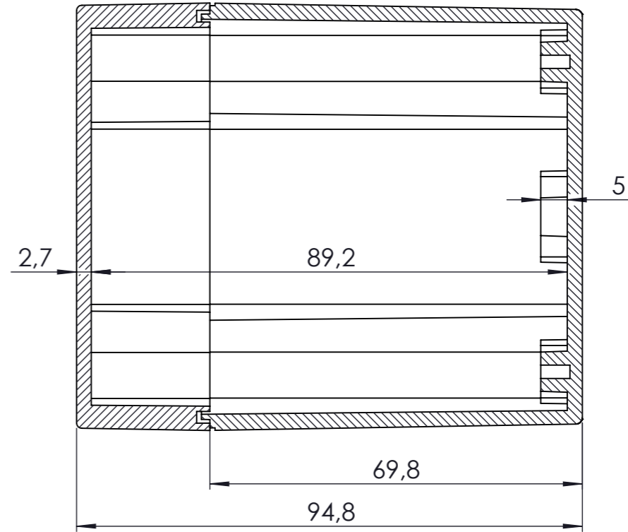
KESIT A-A
