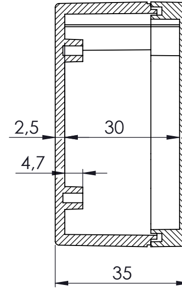
KESIT A-A
