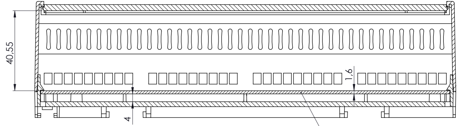
KESIT A-A
