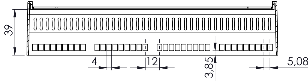
KESİT A-A
