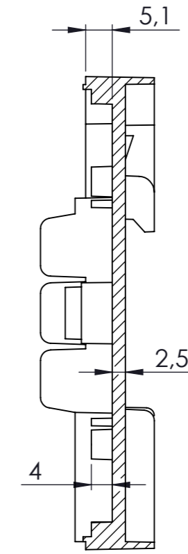
KESİT A-A
