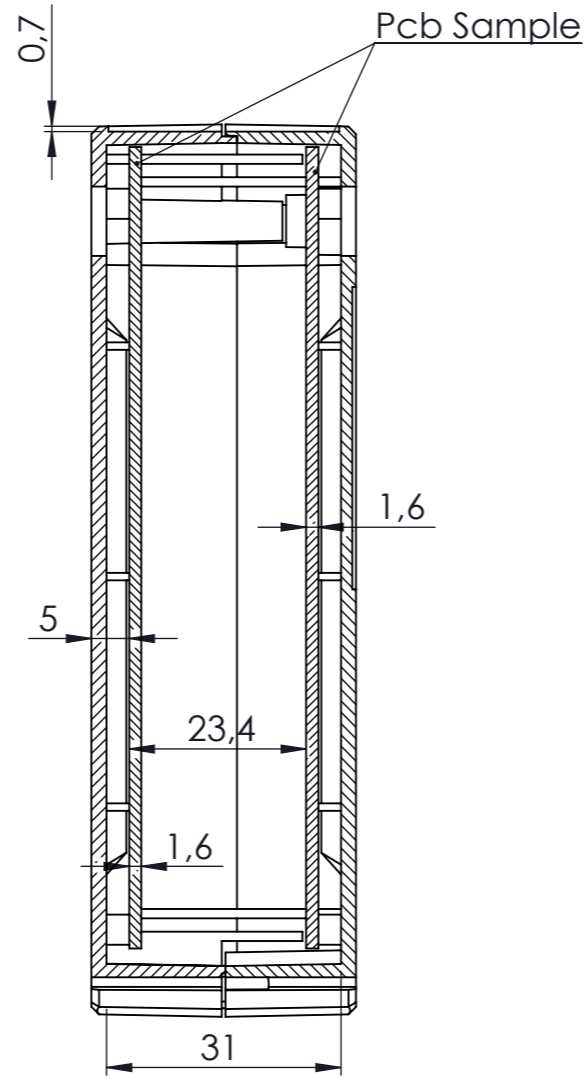
KESIT A-A
