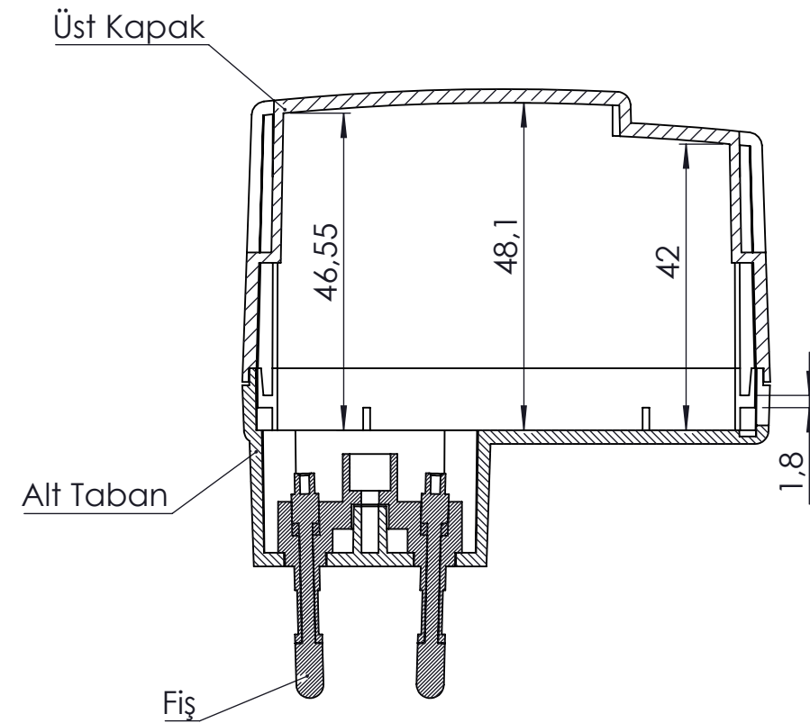
KESİT A-A
